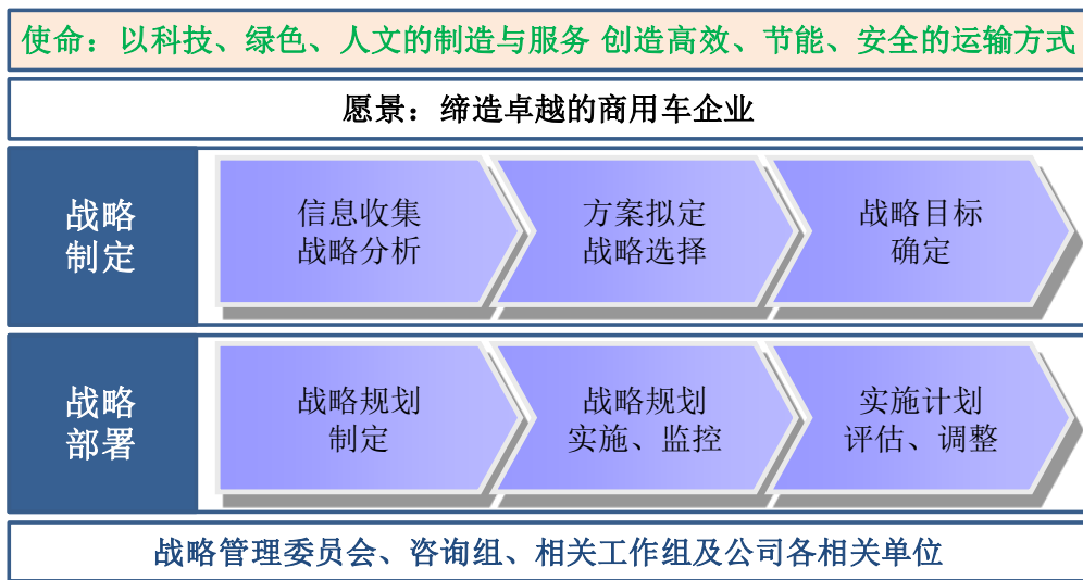
图 4 战略管理图
